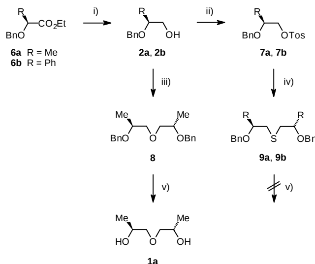
Scheme 3 Preparation of \text{C}_2 -symmetric diglycole 1a . Reagents, conditions, and yields: i) \text{LiAlH}_4 , THF, 23 °C, 90 min, 2a : 98%, 2b : 86%; ii) \text{TosCl} , pyridine, 23 °C, 16 h, 7a : 94%, 7b : 93%; iii) + 7a , NaH, DMF, 50 °C, 3 h, 8 : 73%; iv) \text{Na}_2\text{S} , 16 h, 9a : DMF, 50 °C, 92%, 9b : acetone, 70 °C, 85%; v) Pd–C, \text{H}_2 (1 bar), EtOH, 23 °C, 16 h, 1a : 90%
